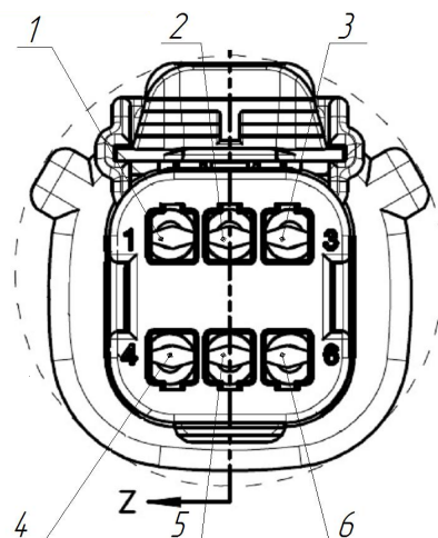
Рис. 4. Вид на разъем кабельной трассы ДУТ.
